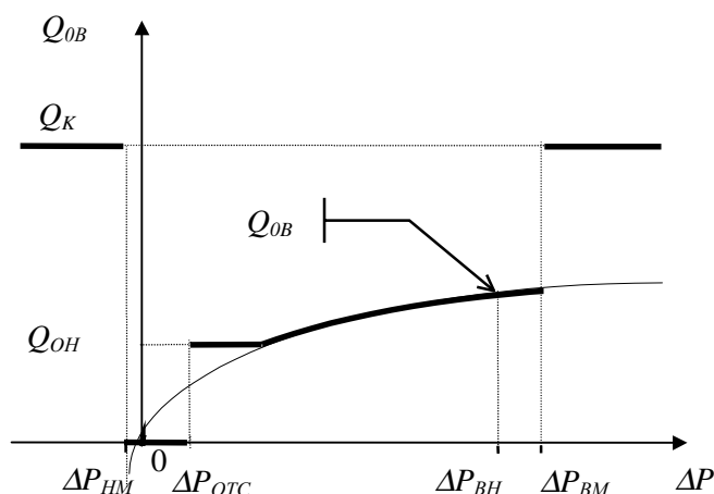
Рисунок 2.7 Вычисление объемного расхода по значениям перепада давления
