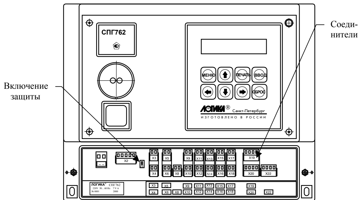
Рисунок 3.2 Корректор СПГ762. Вид спереди
