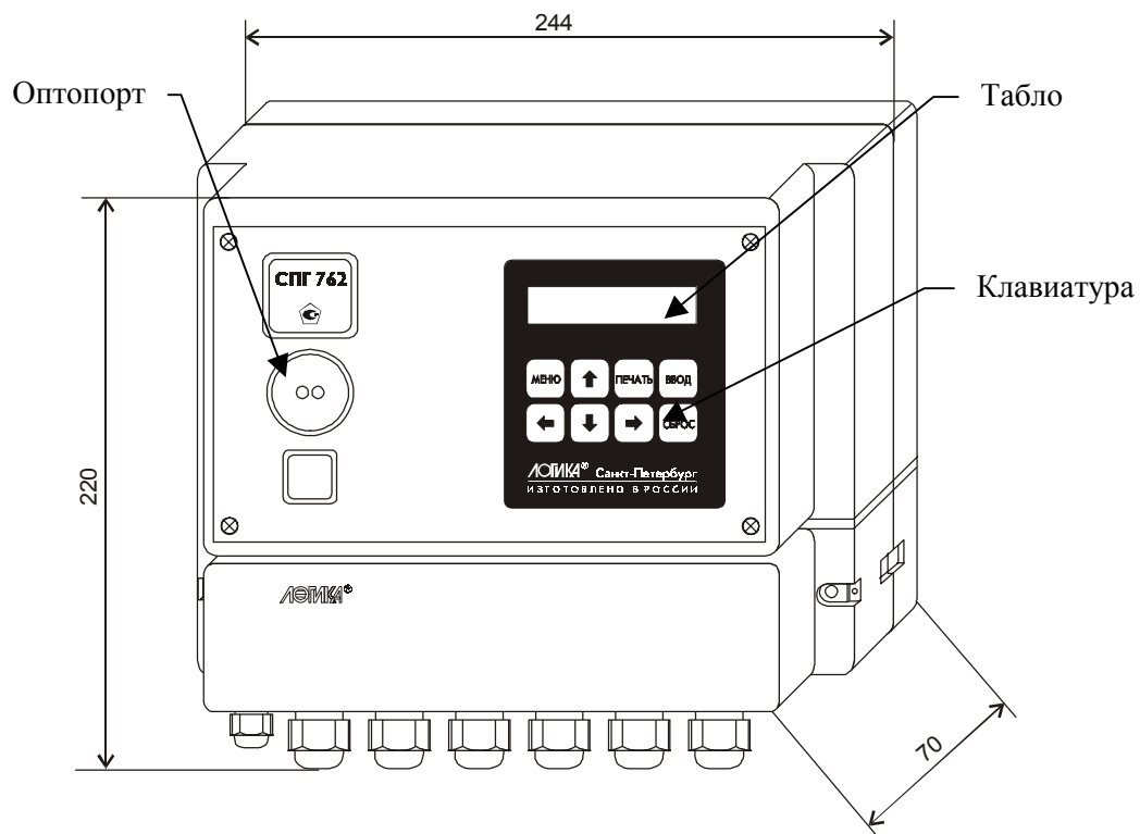
Рисунок 3.1 Внешний вид корректора СПГ762
